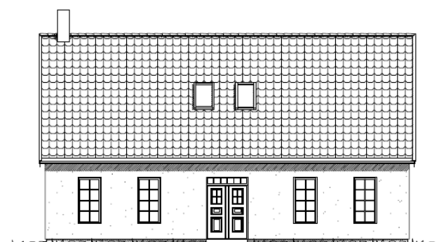
FASAD MOT SYDÖST
